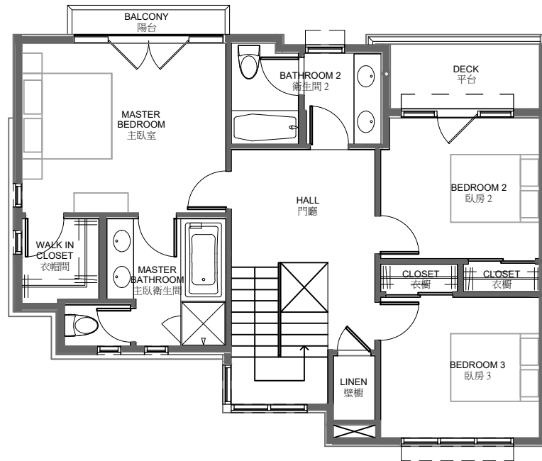
Second Floor Plan 997 S.F. 二樓平面圖
