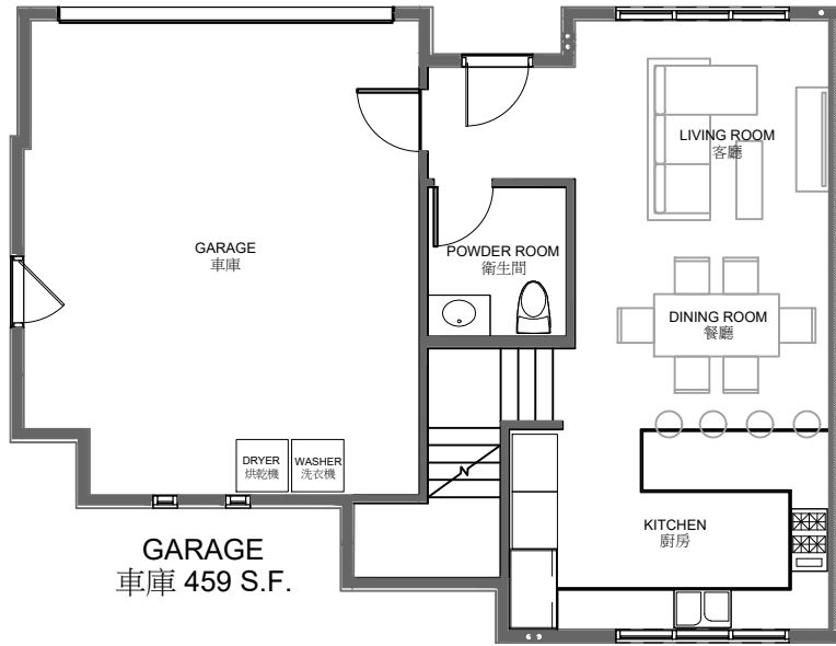
First Floor Plan 528 S.F. 一樓平面圖
